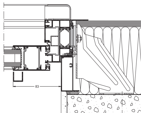
Schüco ASS 41 SC Pose en ITI avec tapées rapportées
