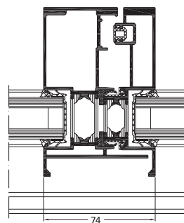
Schüco ASS 41 SC Point 6 réduit 74 mm
