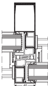
Schüco ASS 41 SC Chicane grande inertie
